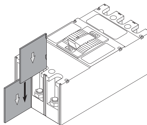
Межполюсные барьеры
