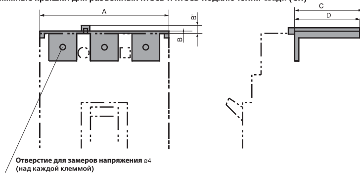
Клеммные крышки для разъёмных МССВ и МССВ подключения сзади (CR)
