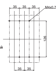
План крепежных отверстий (вид спереди)
