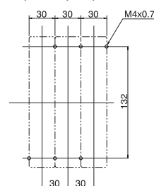
План сверления отверстий (вид спереди)
