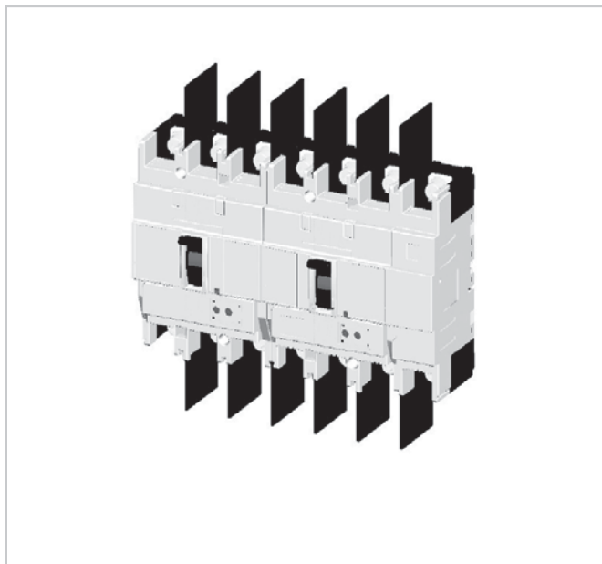
Межполюсные барьеры между смежными автоматическими выключателями МССВ
