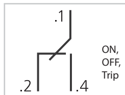
Обозначение контактов и функция дополнительного контакта общего назначения.
