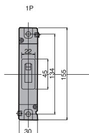
S125-NF – переднее присоединение
