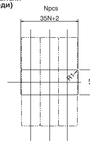
Сечение панели (вид спереди)
