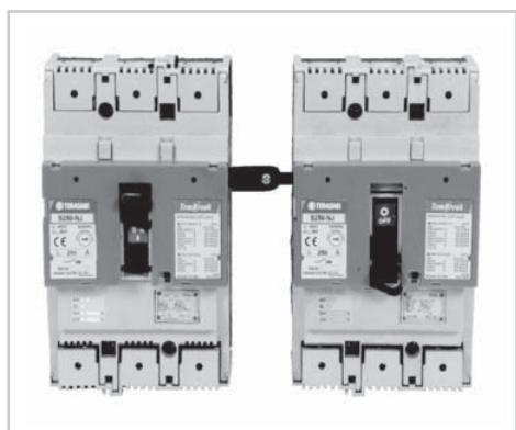
Жесткая взаимоблокировка
